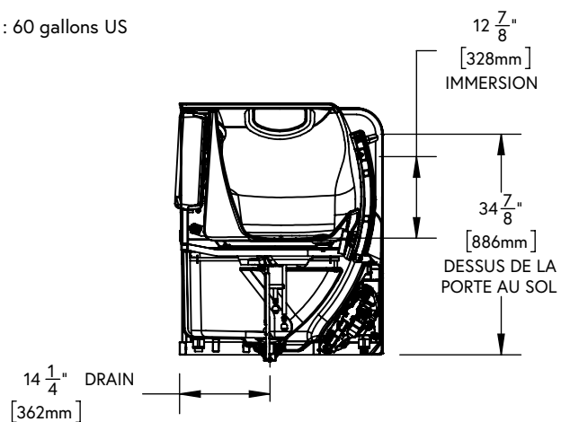
PORTE PLEINE HAUTEUR
