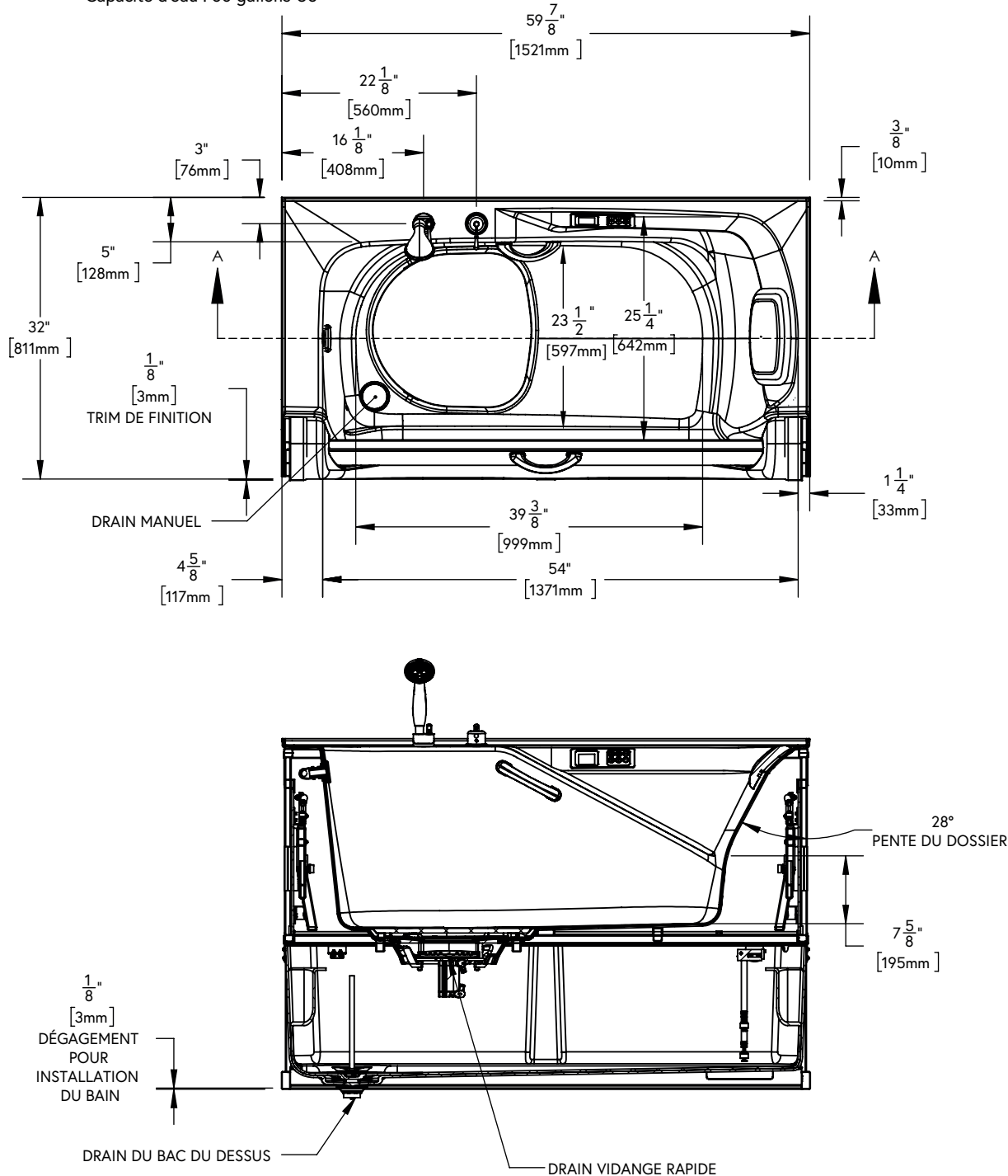
VUE DE COUPE
